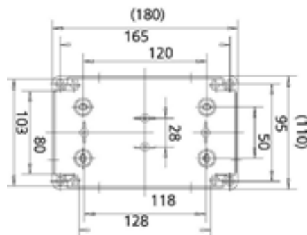
Côtes de perçage pour fixations
